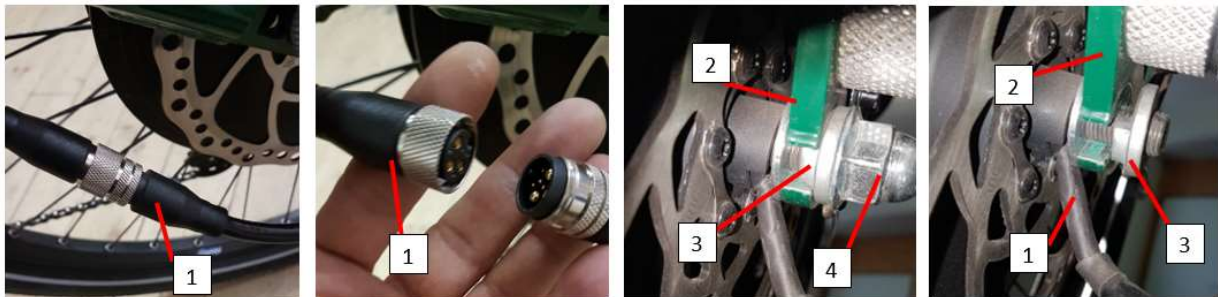
Abbildung 28: Ausbau des Hinterrades
