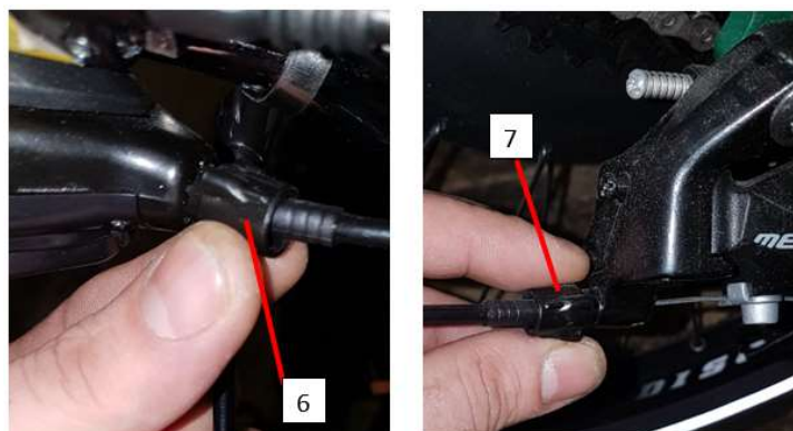
Abbildung 26: Einstellschrauben für Seillänge
