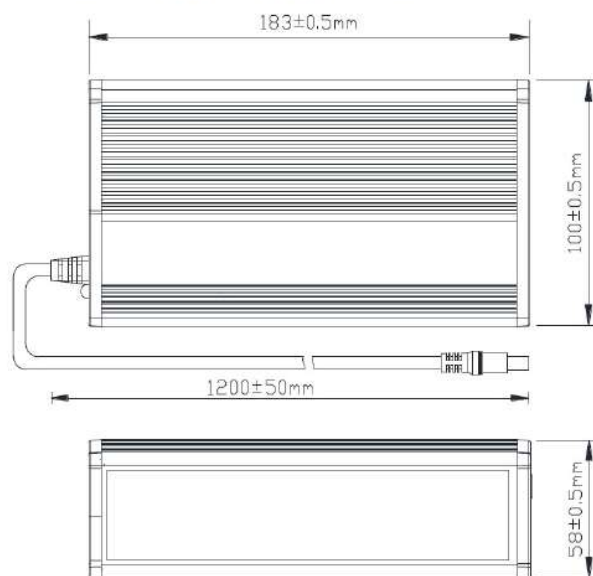
Abbildung 20: Darstellung des Ladegerätes
